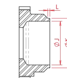
VÁLVULA DE ESFERA DIRECIONAL PASSAGEM REDUZIDA (PR)
